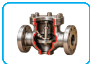
VAN MỘT CHIỀU NÂNG
