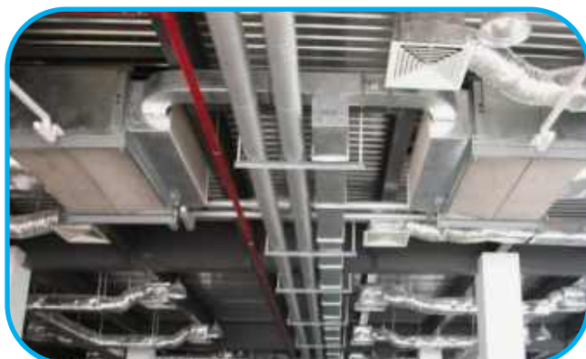
LẮP ĐẶT HỆ THỐNG ĐIỀU HÒA ÂM TRẦN ỐNG GIÓ
